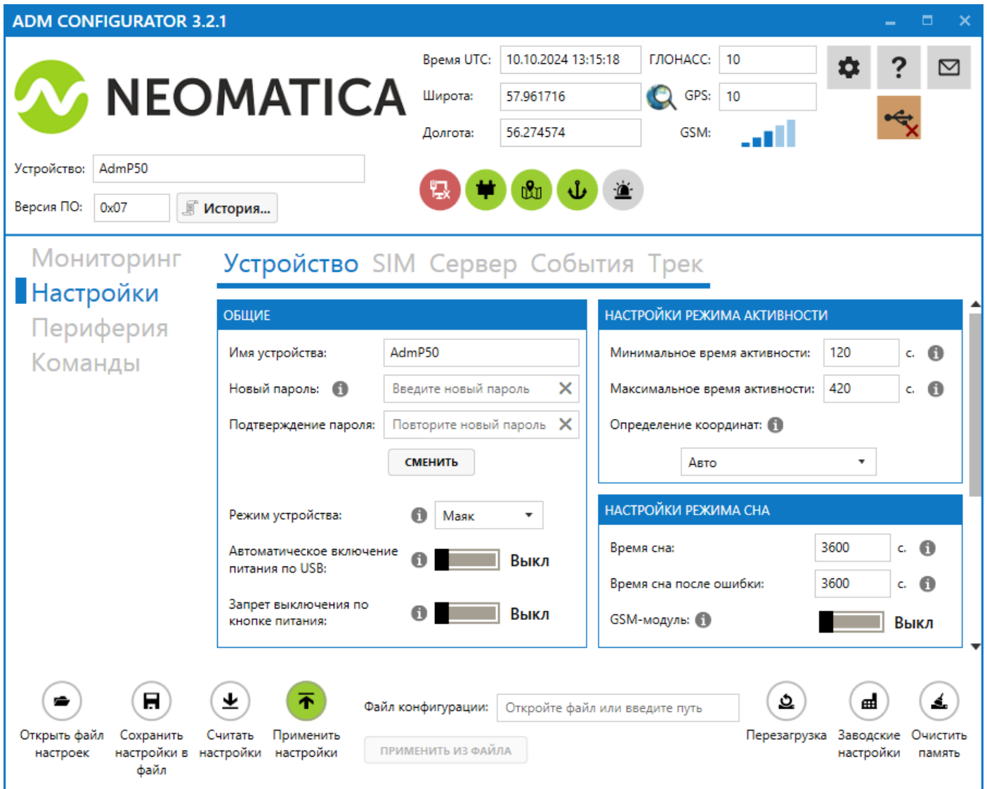
Снимок экрана 4– ADM Configurator: Настройки\Устройство
